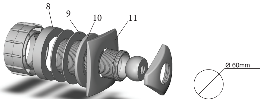
Assemblage sur paroi coque Prefabricated polyester pool assembly Montaje piscina prefabricada de poliester
