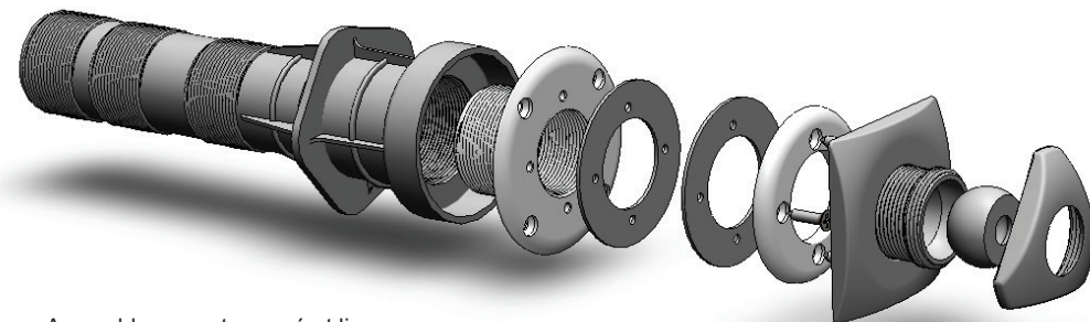
Assemblage sur traversé et liner Assembly with threaded wall conduit and liner Montaje pasamuros roscado y liner
