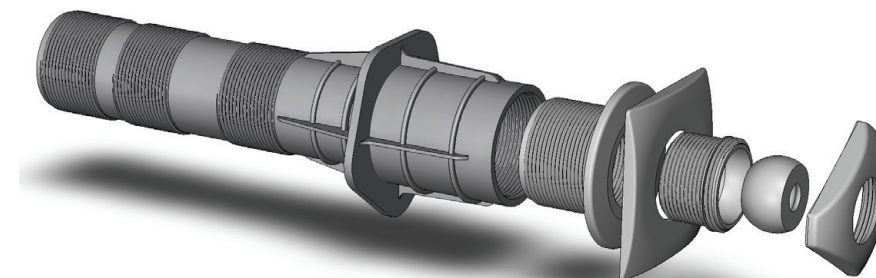
Assemblage sur traversé Assembly with threaded wall conduit Montaje con pasamuros roscado
