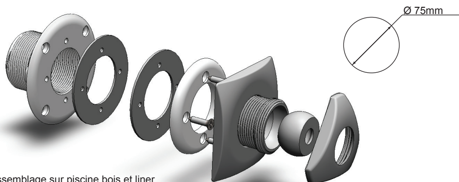
Assemblage sur piscine bois et liner Wooden pool with liner assembly Montaje piscina madera con liner
